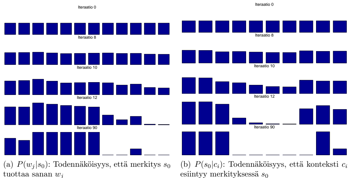
Kuva 1: EM algoritmi. Kuva esittää algoritmin konvergoitumisen. Sanat oikealta vasemmalle lueteltuna: yksi, kaksi, kolme, neljä, viisi, seitsemän, kahdeksan, mänty, leppä, haapa, koivu, kataja. Lauseet ovat samassa järjestyksessä kuin kysymyksessä.
