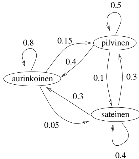
Kuva 1: Säätila Markov-ketjuna
