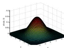
Kuva: Symmetrinen 2D-normaaliijakauma
