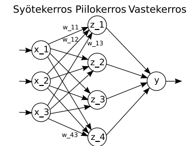
Kuva: Monikerrosperseptroniverkko (MLP) yhdellä ulostulolla.
