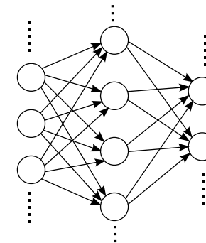
Kuva: Yleinen monikerrosperseptroniverkko (MLP).
