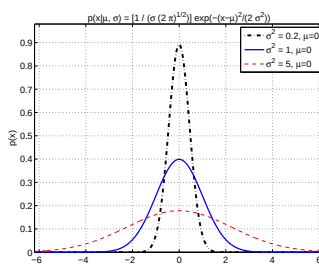
Kuva: Normaalijakauma kolmella eri \sigma :n arvolla
